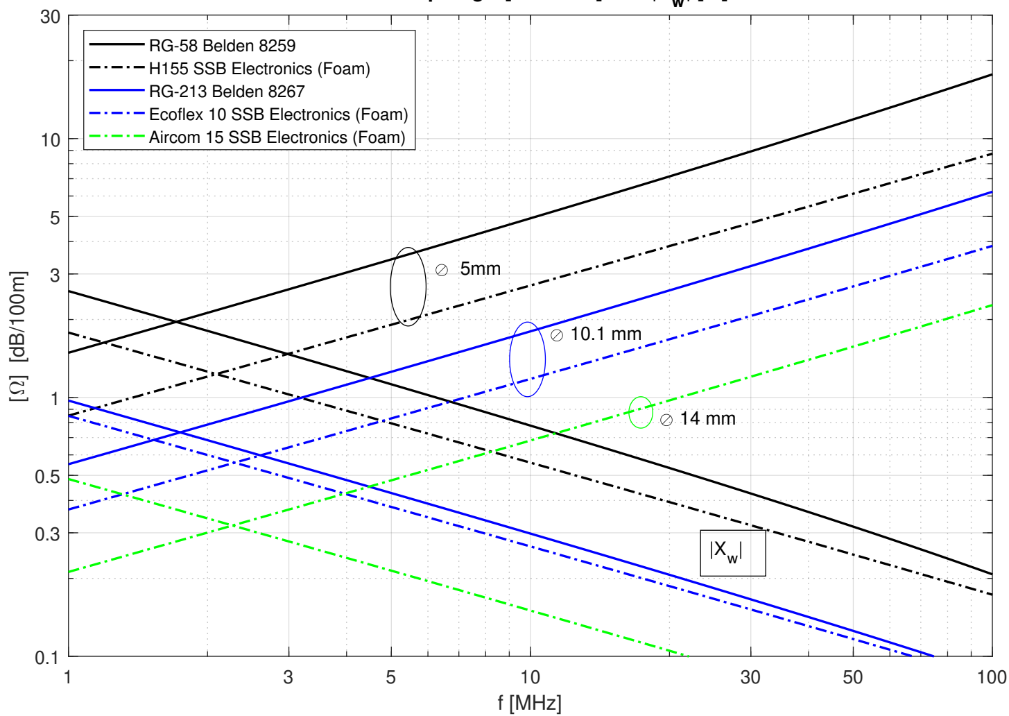
Kabeldämpfung A[dB/100m] und |X_w| [ \Omega ]
